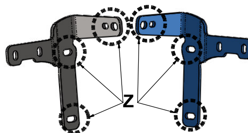
Pieza 2.1 Refuerzo delantero de fijación a la caja L.C.
