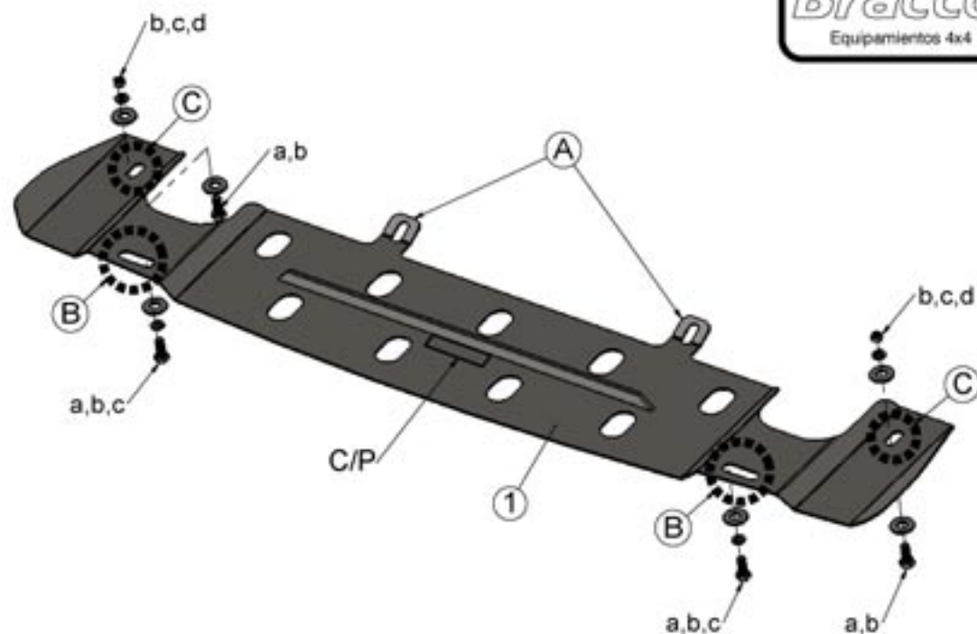
Fig. 1 Vista inferior
